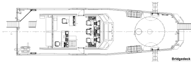
Bridgedeck
