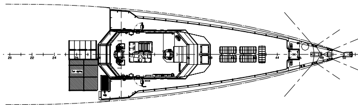
Bridgedeck
